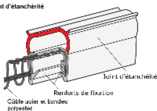
Joint d'étanchéité
